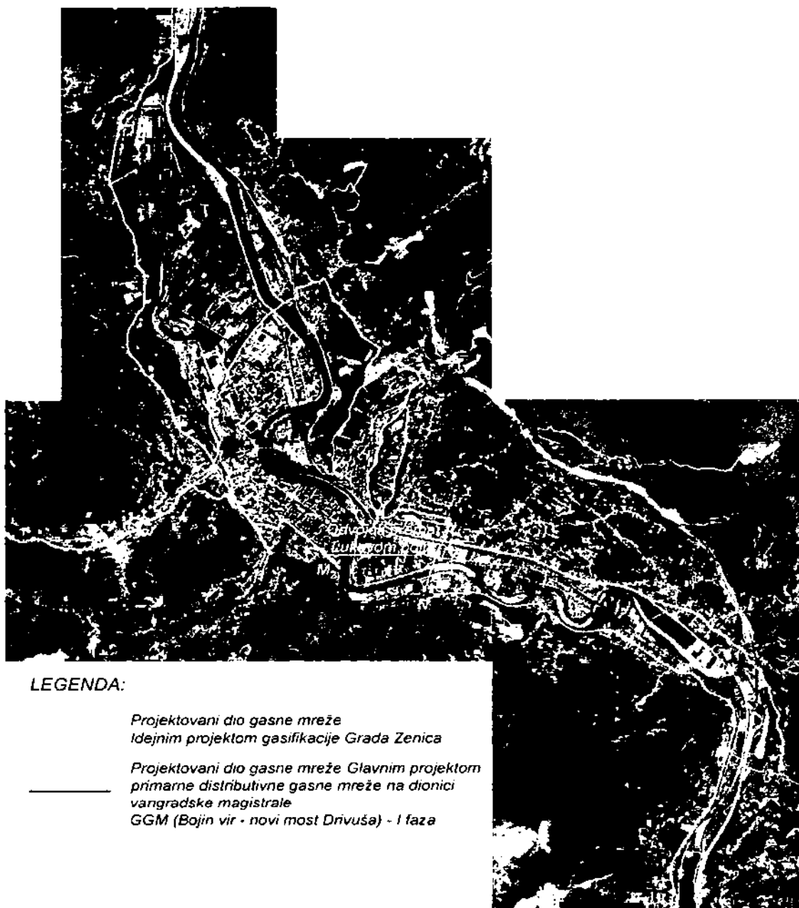
Slika 3. Trasa primarne gasne distributivne mreže na dionici vangradske magistrale GGM (Bojin vir – novi most Drivuša) u Gradu Zenica – I faza
