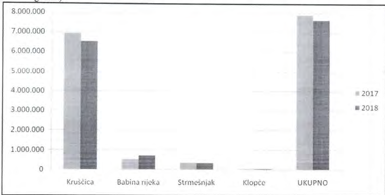
Graf 1: Proizvodnja pitke vode po vodozahvatima (ostvareno u 2017. godini i ostvareno u 2018. godini)
