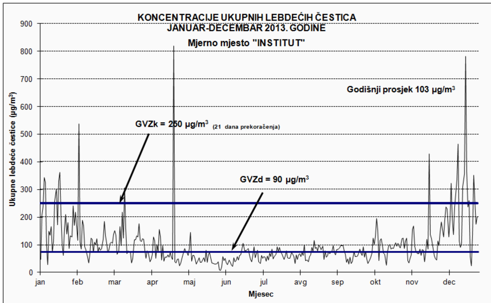
Slika 5. Dnevne koncentracije ukupnih lebdećih čestica za 2013. godinu na mjernom mjestu „INSTITUT“
