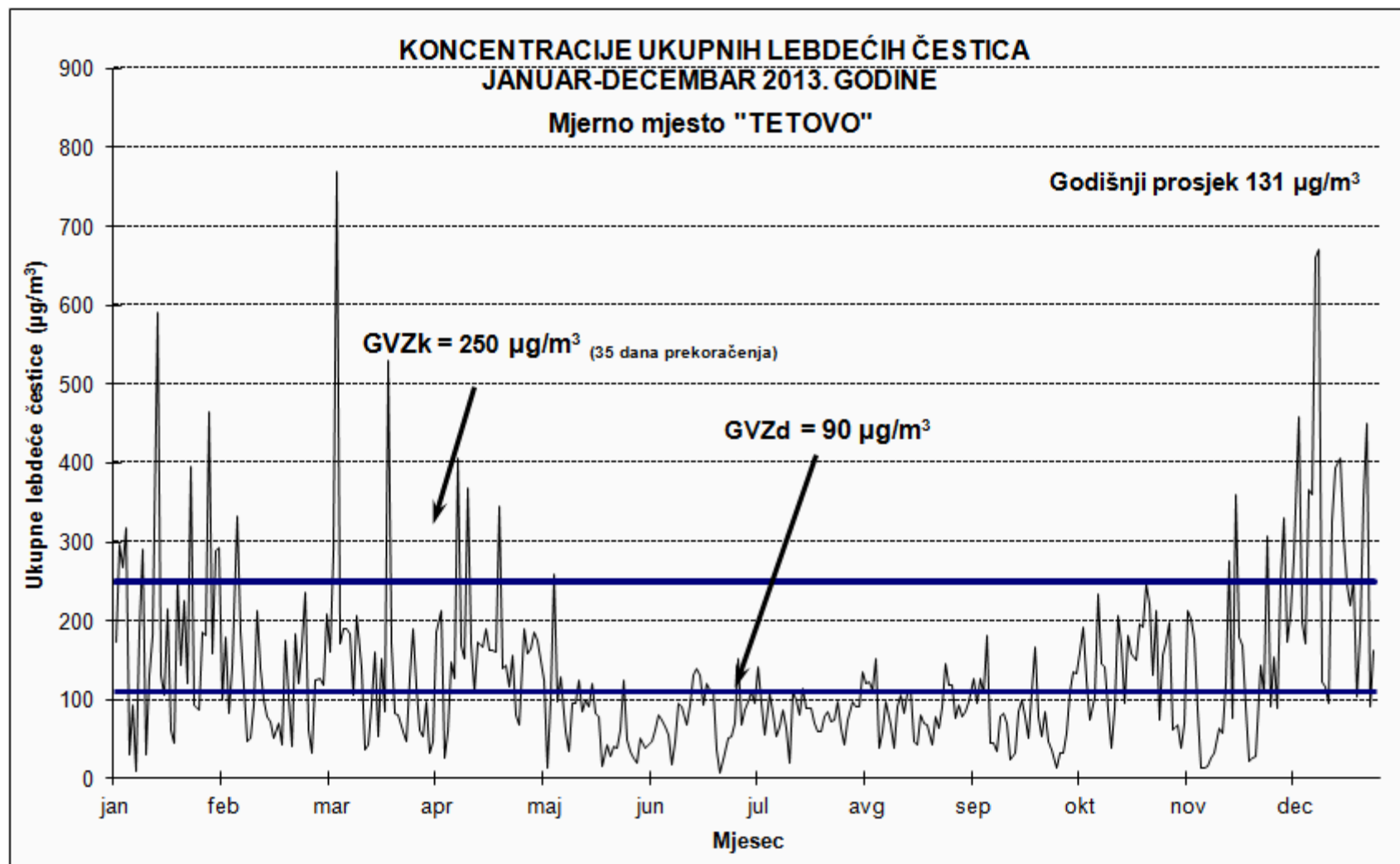
Slika 6. Dnevne koncentracije ukupnih lebdećih čestica za 2013. godinu na mjernom mjestu „TETOVO“
