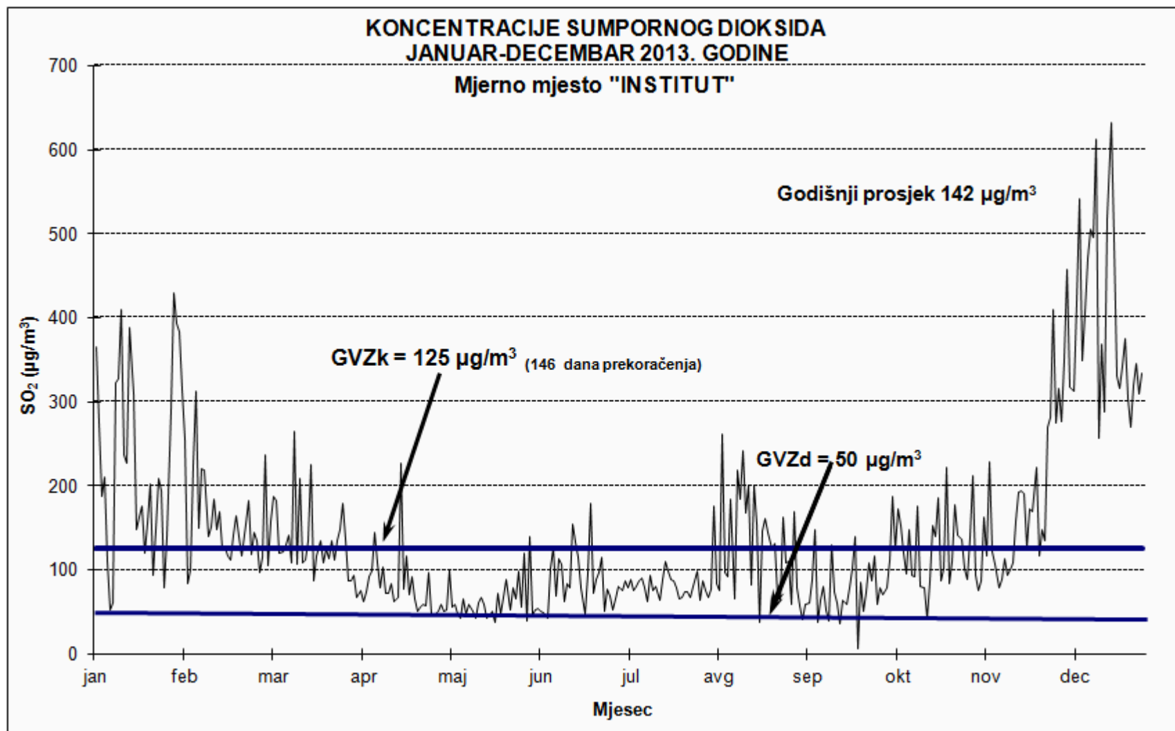
Slika 2. Dnevne koncentracije SO 2 za 2013. godinu na mjernom mjestu „INSTITUT“
