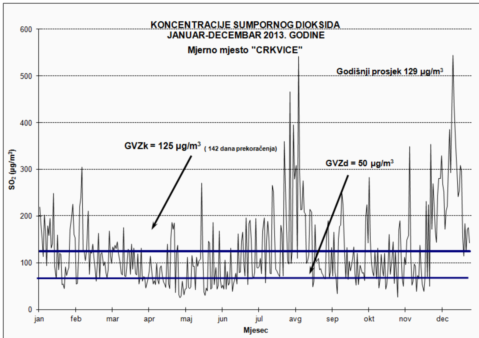
Slika 3. Dnevne koncentracije SO 2 za 2013. godinu na mjernom mjestu „CRKVICE“
