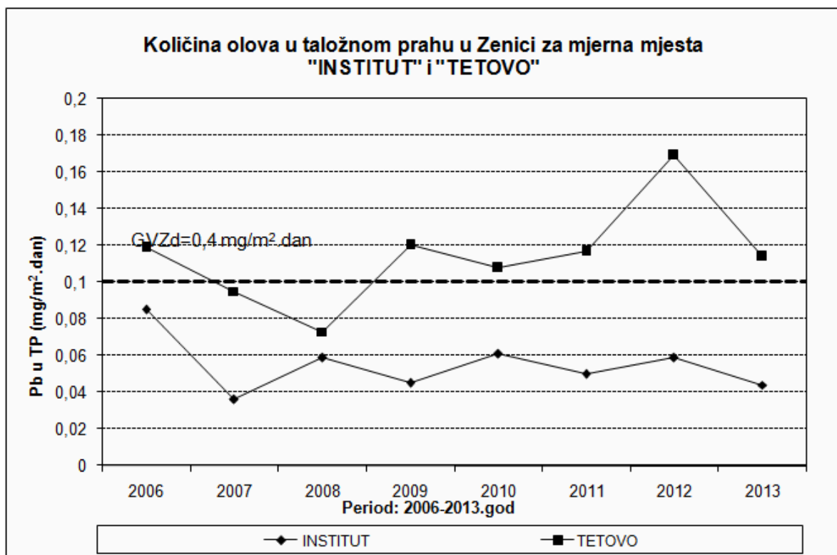
Slika 13. Sadržaj olova u taložnom prahu za period 2006-2013. godina
