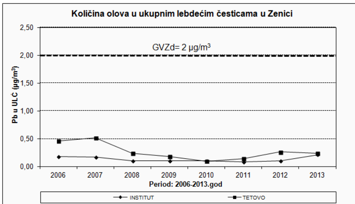
Slika 11. Sadržaj olova u ULČ za period 2006-2013. godina
