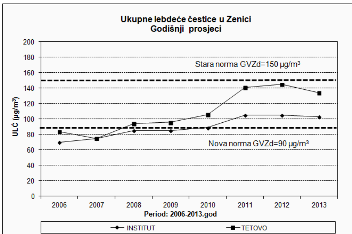
Slika 9. Godišnji prosjeci koncentracija ULČ za period 2006-2013. godina
