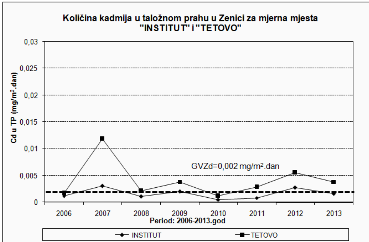
Slika 15. Sadržaj kadmija u taložnom prahu za period 2006-2013. godina
