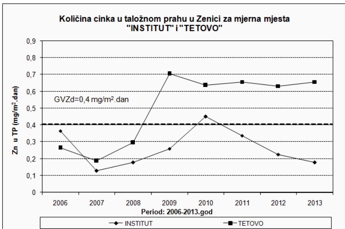
Slika 14. Sadržaj cinka u taložnom prahu za period 2006-2013. godina
