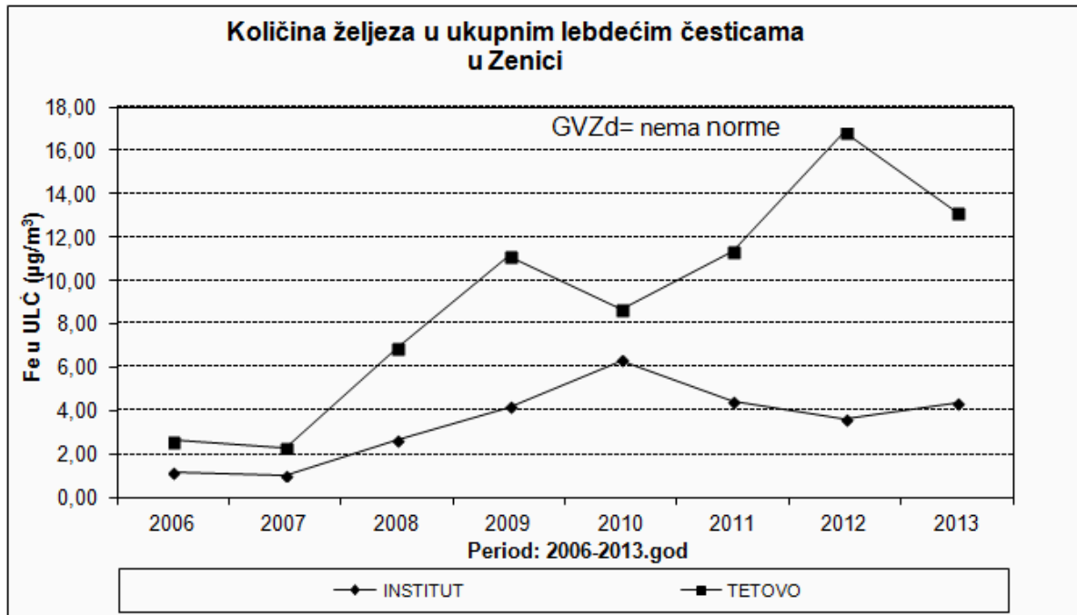
Slika 13. Sadržaj željeza u ULČ za period 2006-2013. godina
