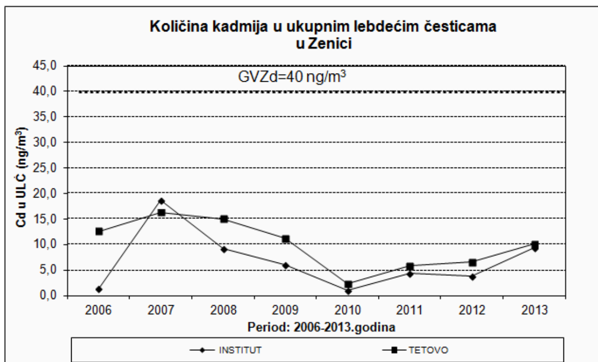
Slika 12. Sadržaj kadmija u ULČ za period 2006-2013. godina
