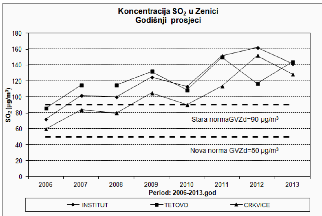
Slika 7. Godišnji prosjeci koncentracija SO 2 za period 2006-2013. godina
