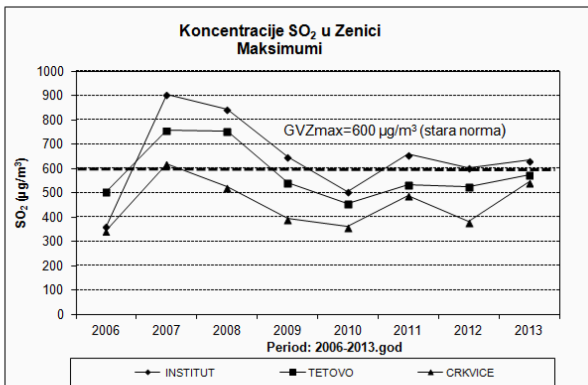
Slika 8. Maksimumi koncentracija SO 2 za period 2006-2013. godina
