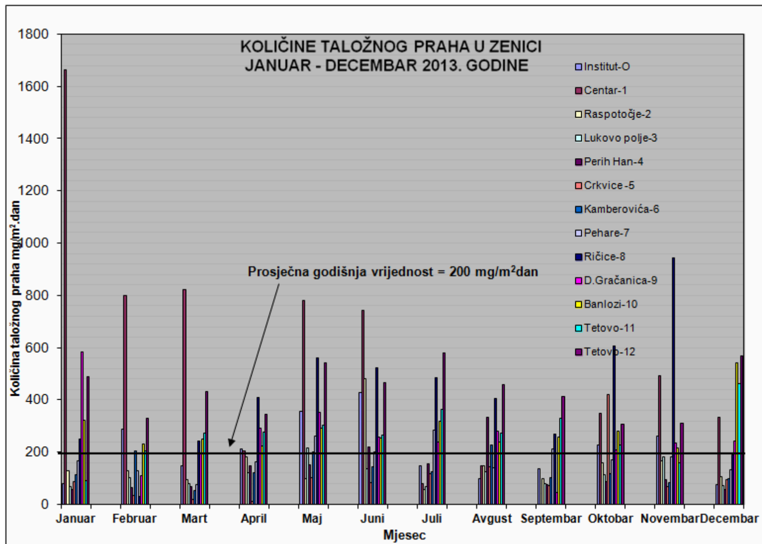
Slika 17. Količina taložnog praha u 2013. godini
