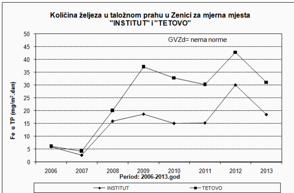
Slika 16. Sadržaj željeza u taložnom prahu za period 2006-2013. godina
