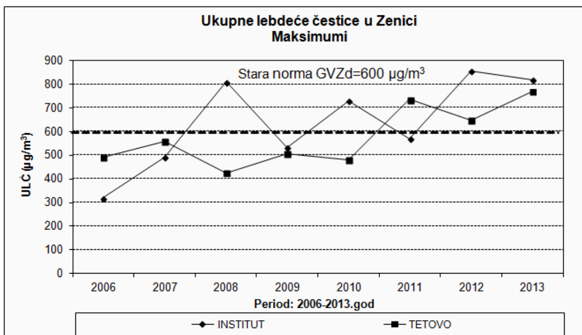
Slika 10. Maksimumi koncentracija ULČ za period 2006-2013. godina
