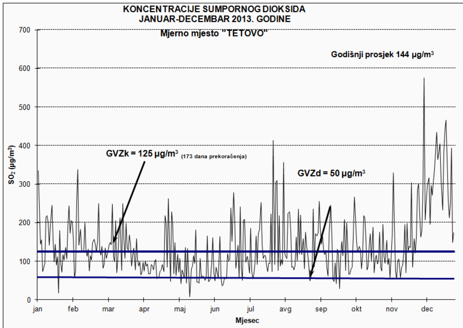
Slika 4. Dnevne koncentracije SO 2 za 2013. godinu na mjernom mjestu „TETOVO“
